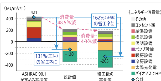
本施設における一次エネルギー消費量
