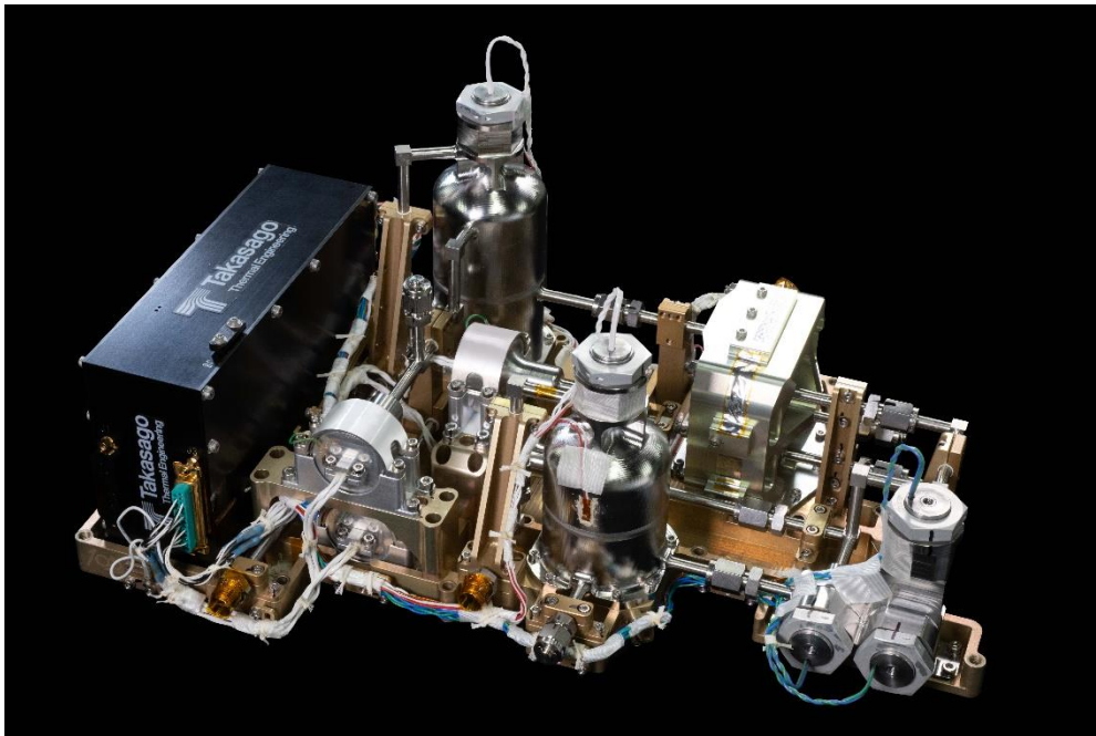
月面用水電解装置 外観
