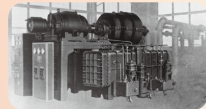
高砂荏原式ターボ冷凍機
