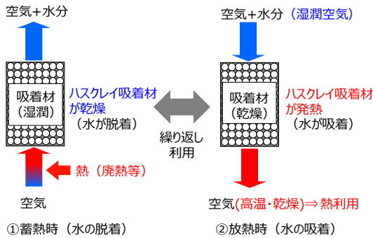
蓄熱材の原理
